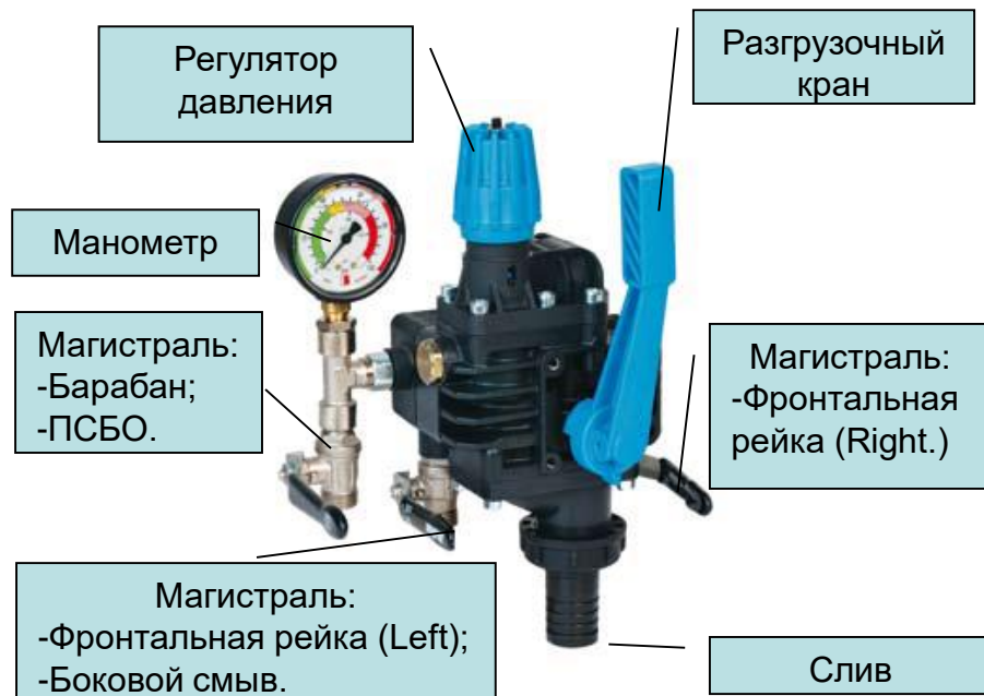
Рис. 26 Блок управления.
