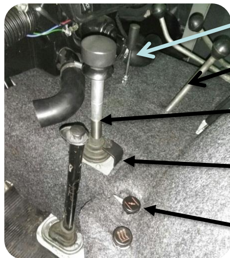
Рис.4. Система рычагов.
