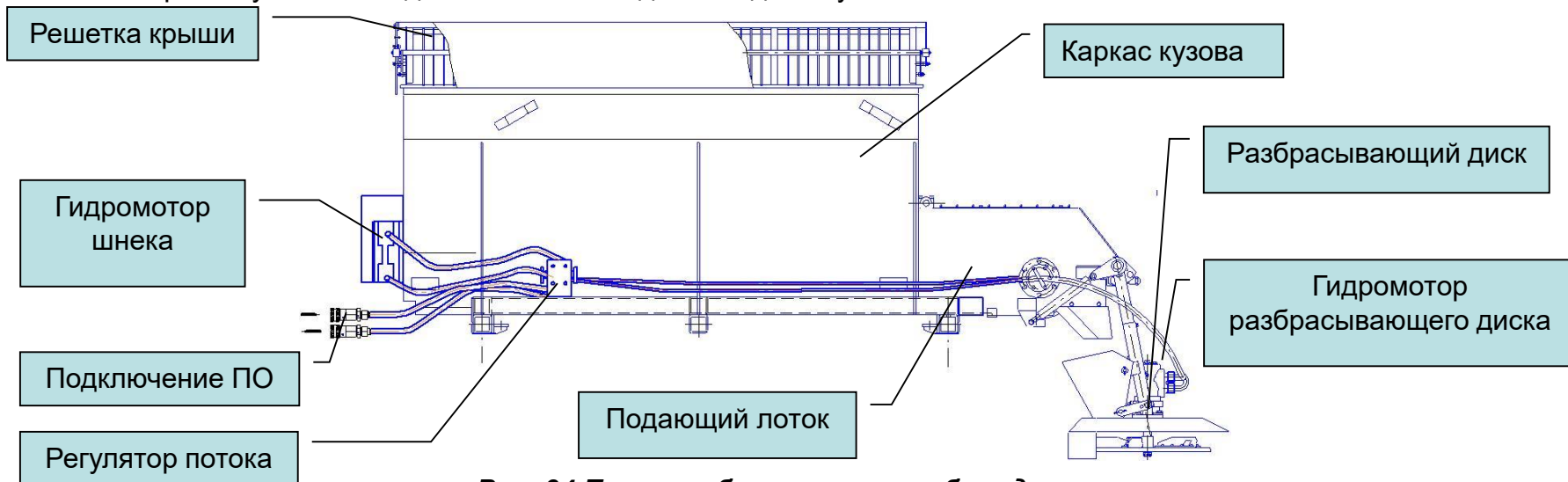
Рис. 34 Пескоразбрасывающее оборудование.
