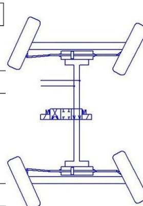
Рис.12. Режим 3. Синхронный режим.
