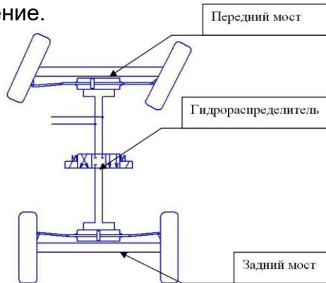
Рис.11. Режим.2. Режим управления только передними колесами.
