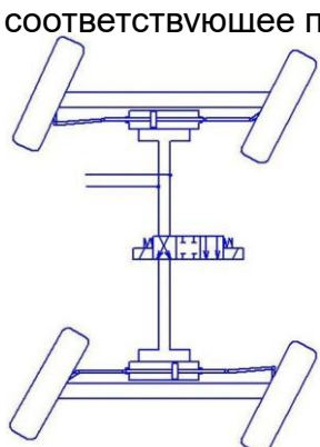
Рис.10. Режим 1. Крабо́вый режим.
