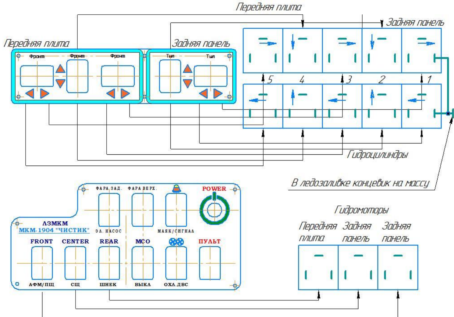
Рис.43 Электрическая схема подключения.
