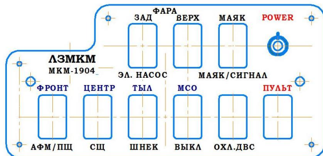
Рис.8. Основной пульт.
