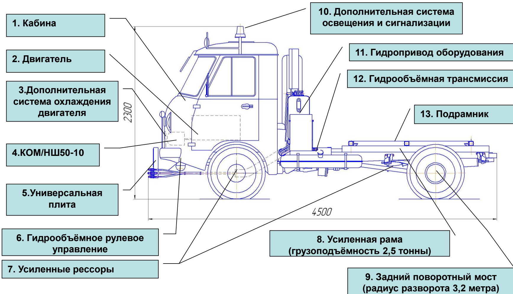
Рис.1. Устройство машины.
