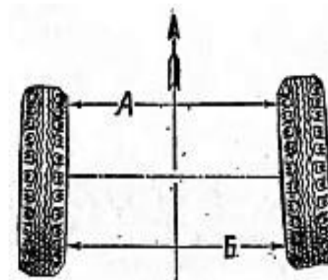
Схождение колес
