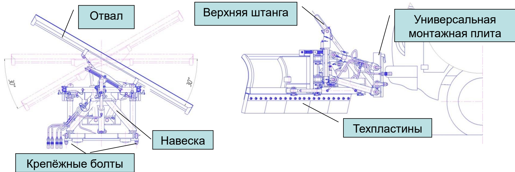
Рис. 30 Отвал поворотный.
