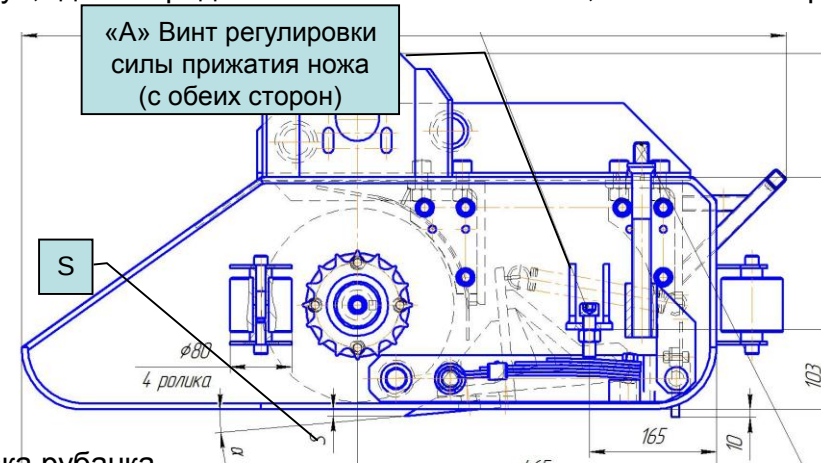
Рис. 41 Регулировка рубанка.
