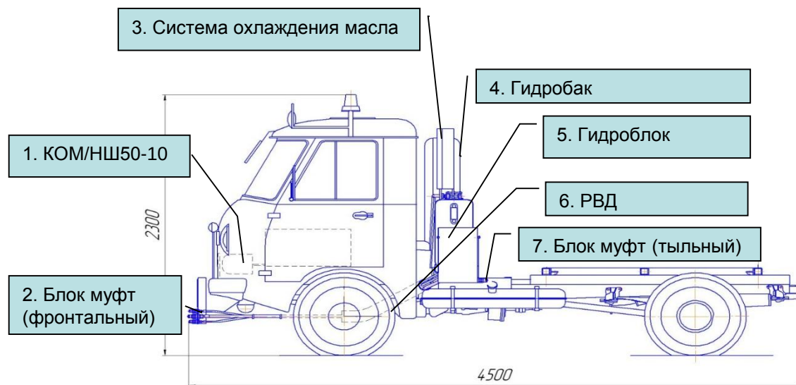
Рис. 16. Гидропривод оборудования:
