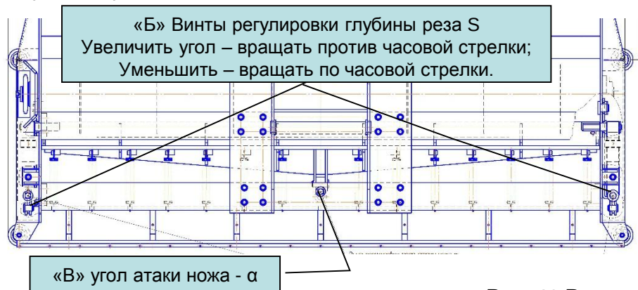
Рис. 41 Регулировка рубанка.
