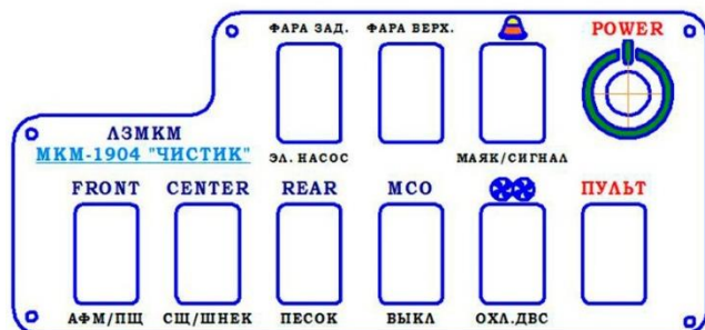
Рис.8. Основной пульт.
