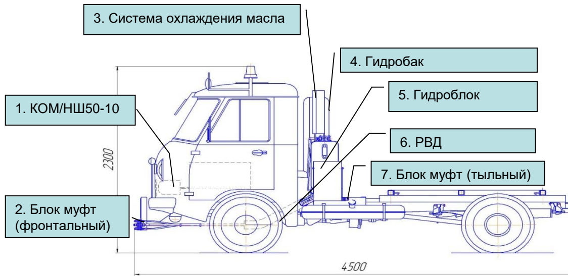
Рис. 16. Гидропривод оборудования:
