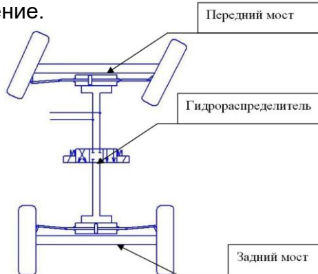
Рис.11. Режим.2. Режим управления только передними колесами.
