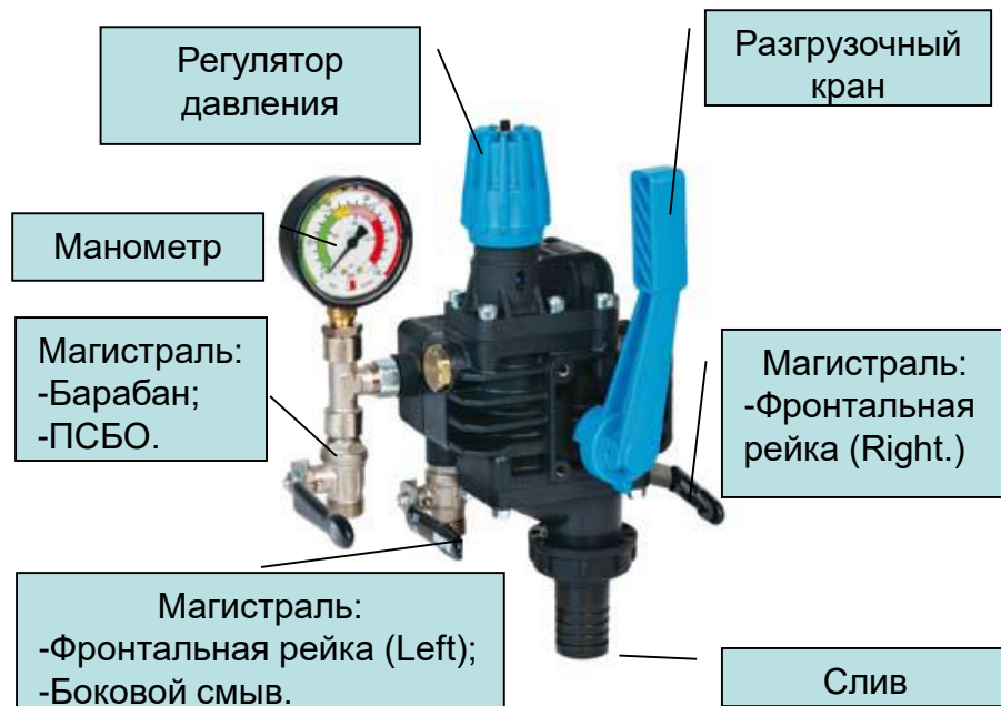
Рис. 26 Блок управления.
